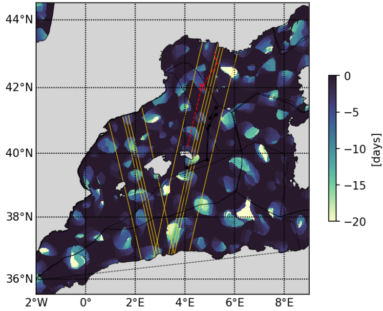
20230517 Retention parameter
