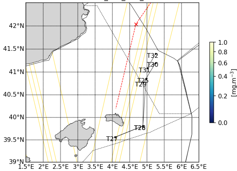
20230516_CLS_CHL_10d
