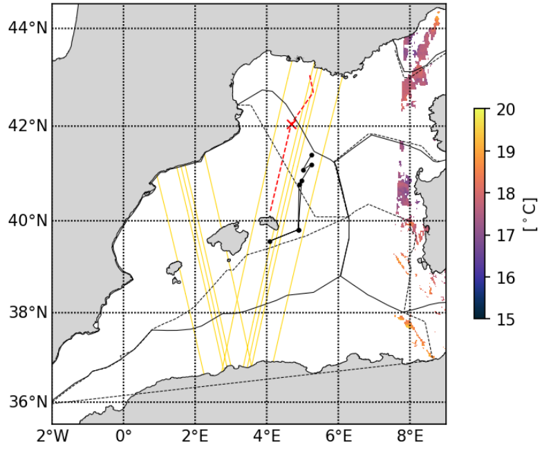
20230516_CLS_SST
