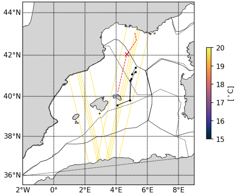
20230515_CLS_SST_7d
