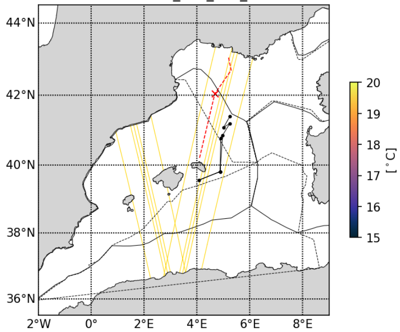
20230515_CLS_SST_5d
