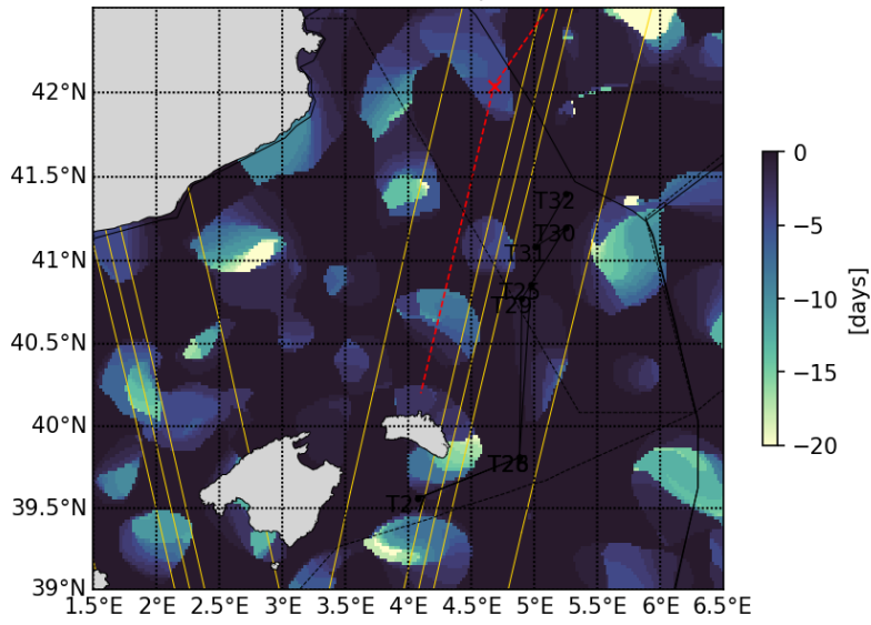
20230517 Retention parameter
