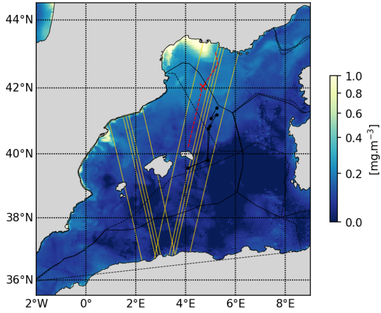
20230515_Copernicus_CHL_L4
