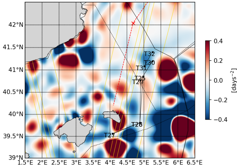
20230517 Okubo-Weiss parameter
