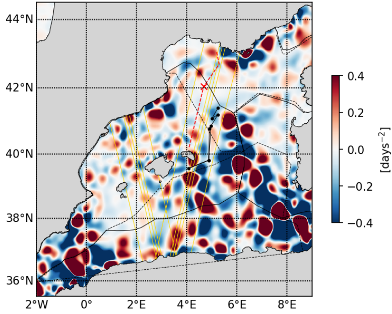
20230517 Okubo-Weiss parameter
