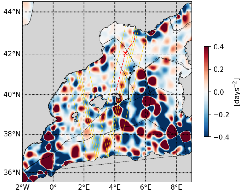
20230515 Okubo-Weiss parameter
