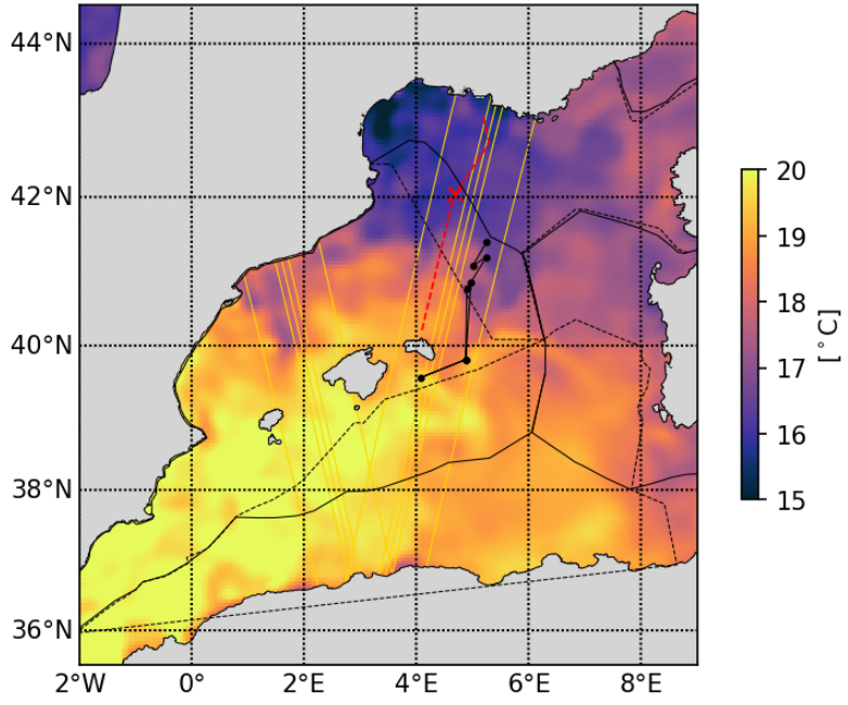
20230514_Copernicus_SST_L4
