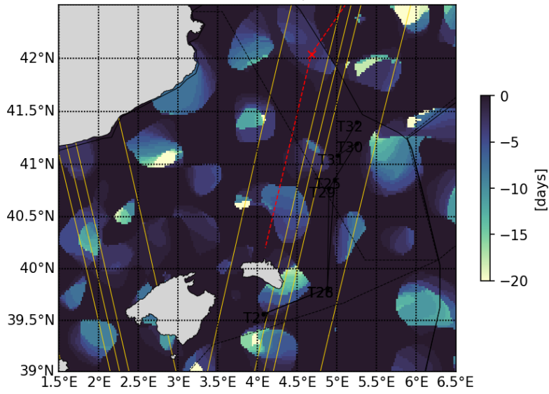
20230515 Retention parameter
