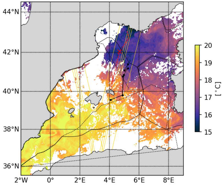
20230514_CLS_SST
