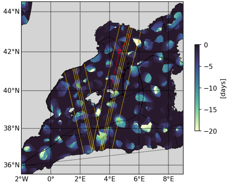
20230515 Retention parameter
