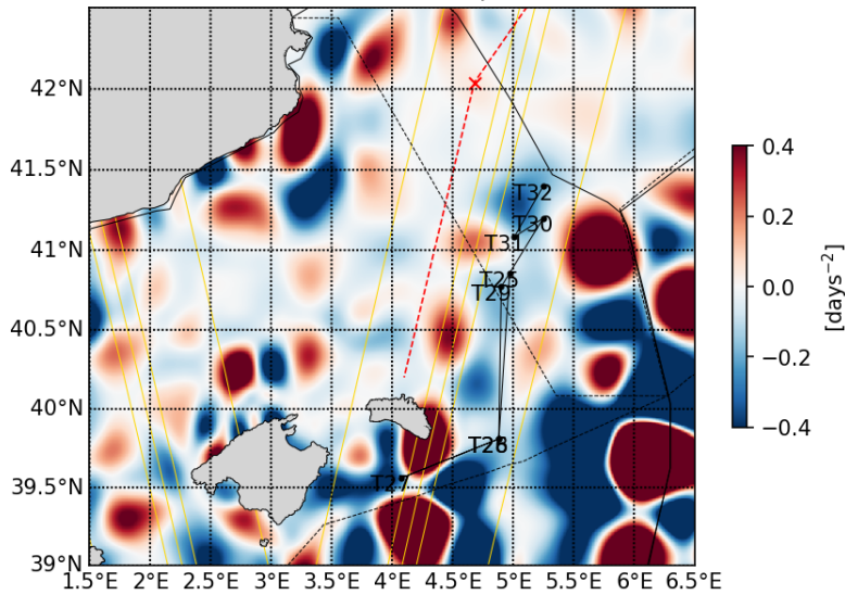
20230515 Okubo-Weiss parameter
