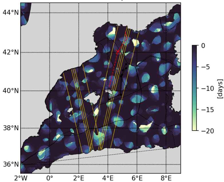
20230514 Retention parameter
