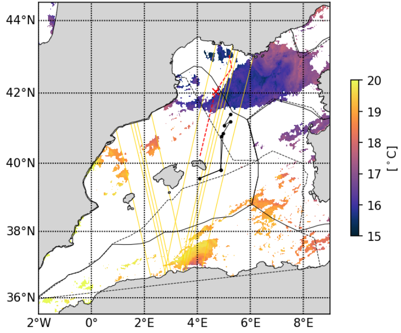
20230513_CLS_SST
