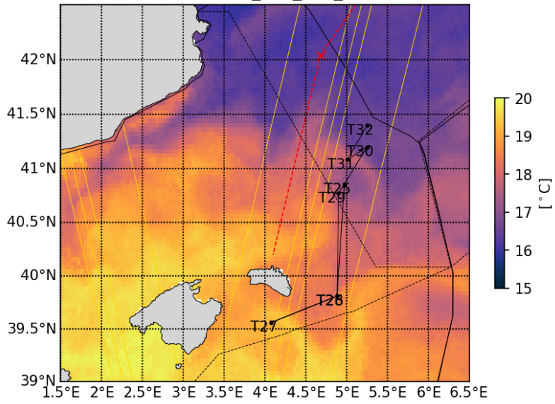
20230512_CLS_SST_7d
