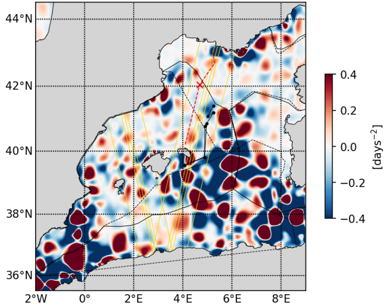
20230514 Okubo-Weiss parameter
