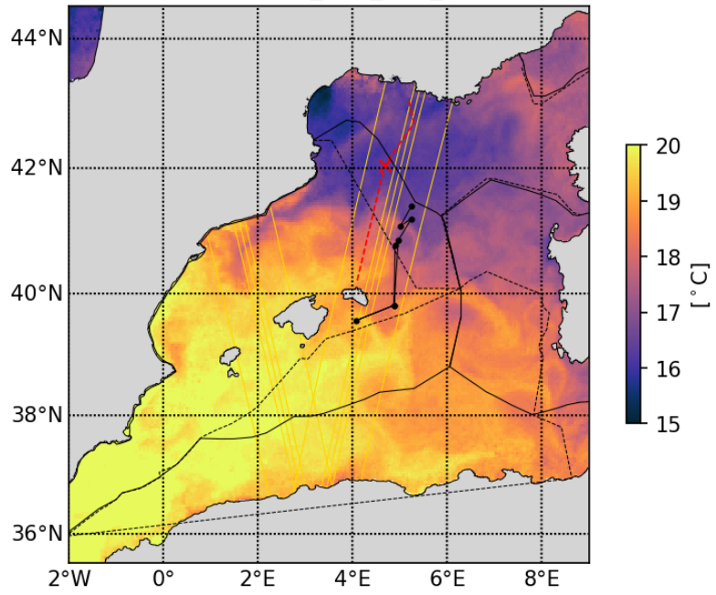
20230512_CLS_SST_7d
