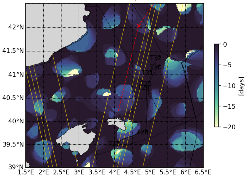
20230514 Retention parameter
