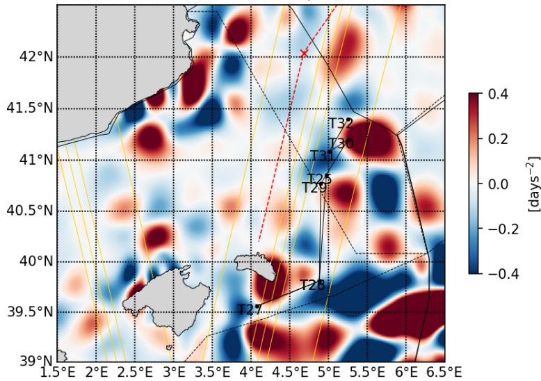
20230510 Okubo-Weiss parameter
