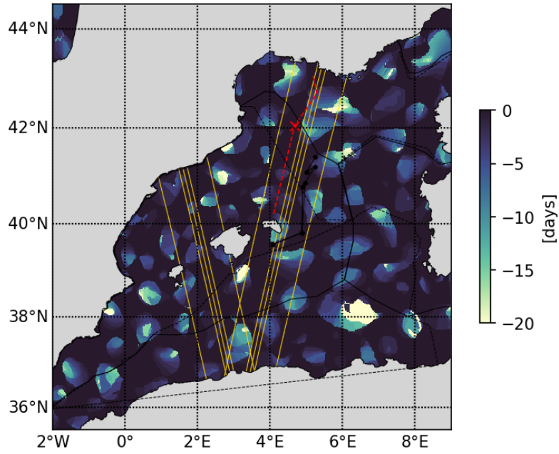
20230510 Retention parameter
