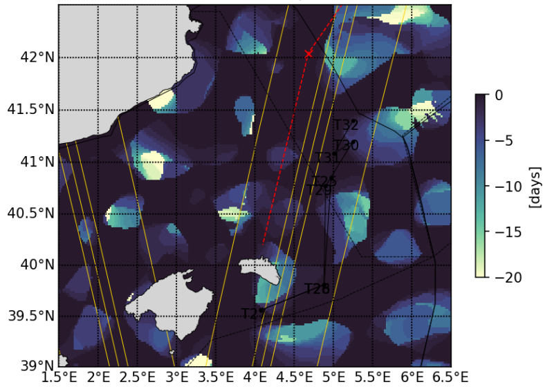
20230510 Retention parameter
