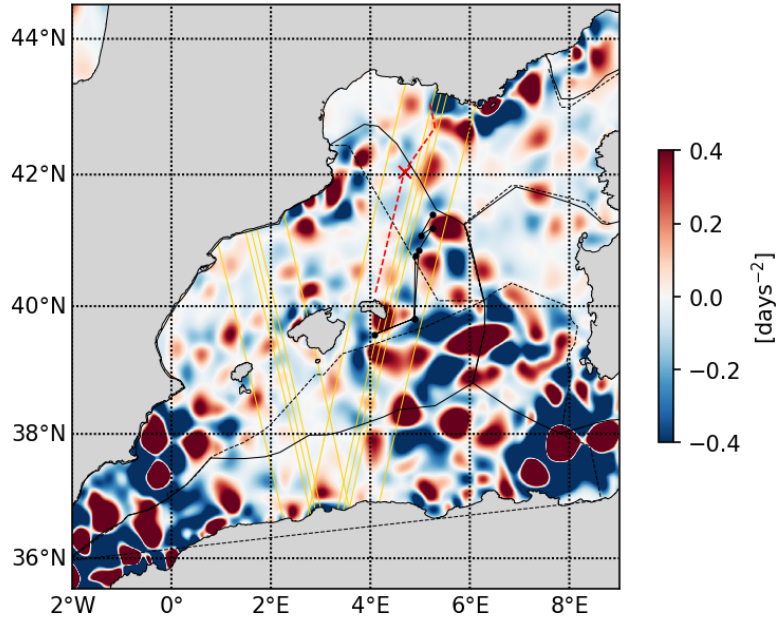
20230510 Okubo-Weiss parameter
