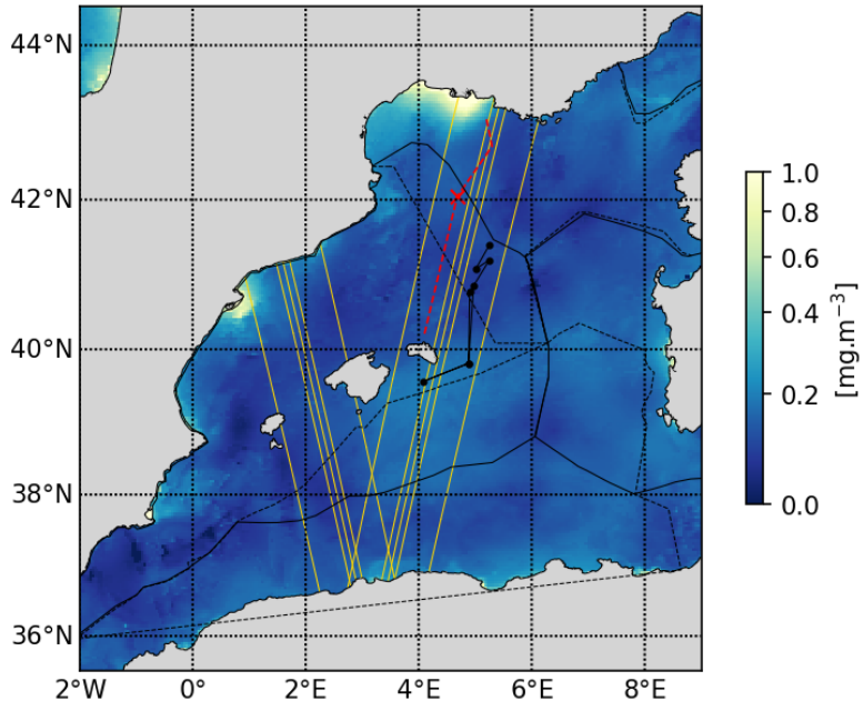
20230507_Copernicus_CHL_L4
