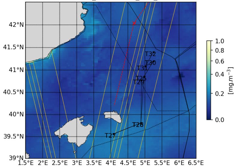
20230507_Copernicus_CHL_L4
