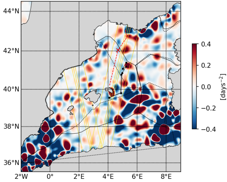
20230509 Okubo-Weiss parameter
