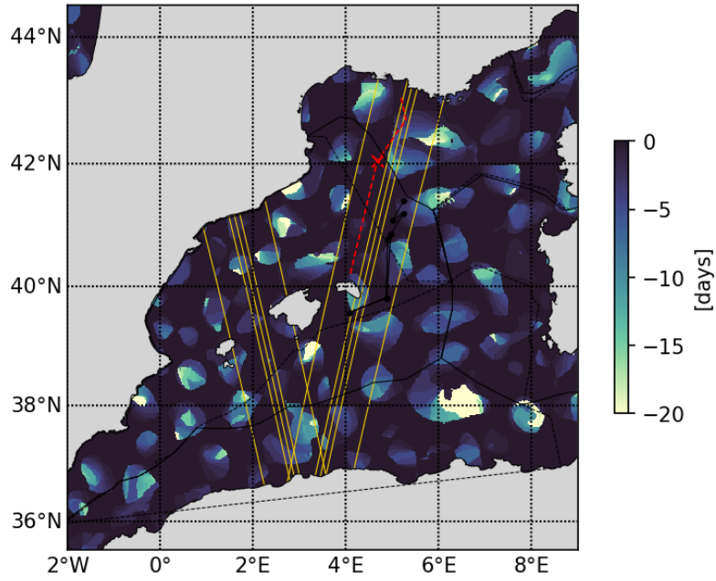
20230509 Retention parameter
