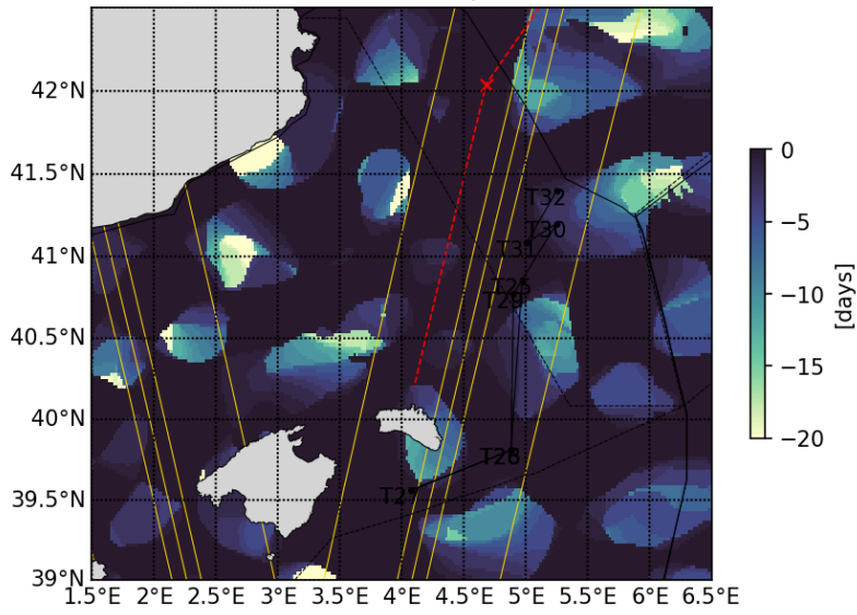
20230509 Retention parameter
