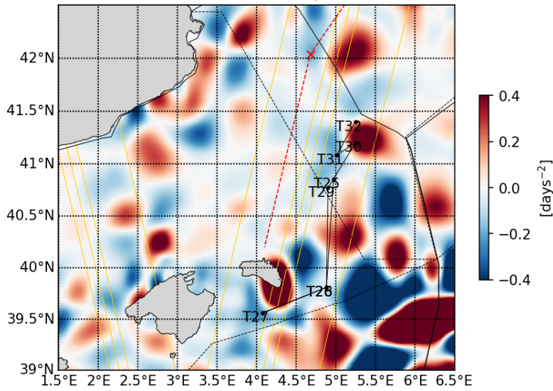
20230509 Okubo-Weiss parameter
