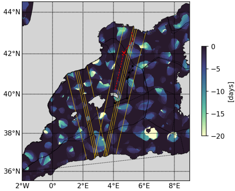
20230508 Retention parameter
