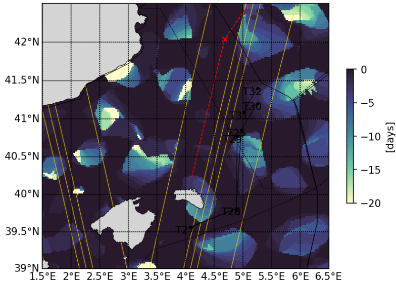
20230508 Retention parameter
