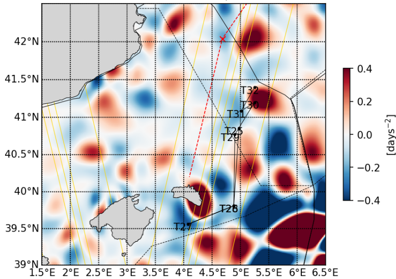
20230508 Okubo-Weiss parameter
