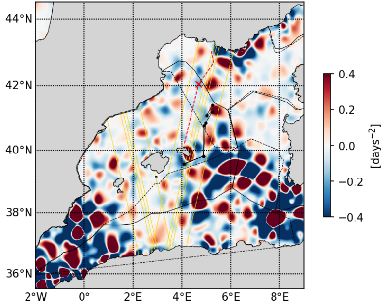
20230508 Okubo-Weiss parameter
