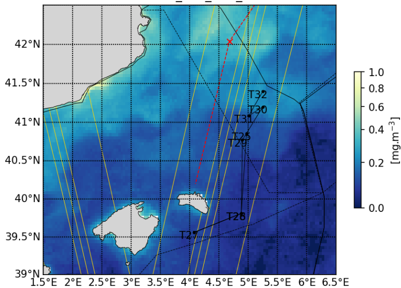
20230507_CLS_CHL_10d
