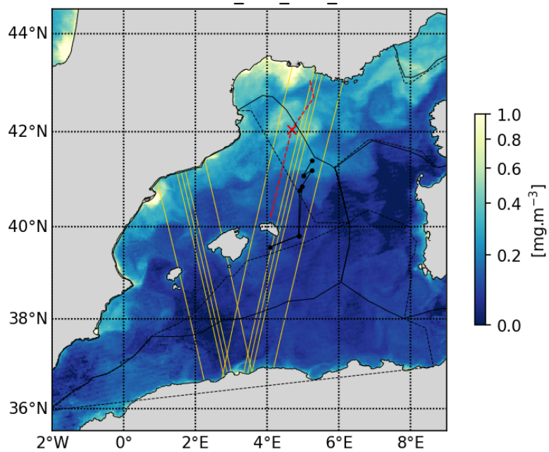
20230505_CLS_CHL_5d
