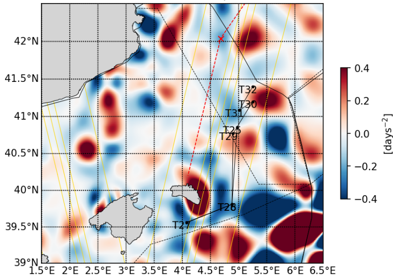
20230507 Okubo-Weiss parameter
