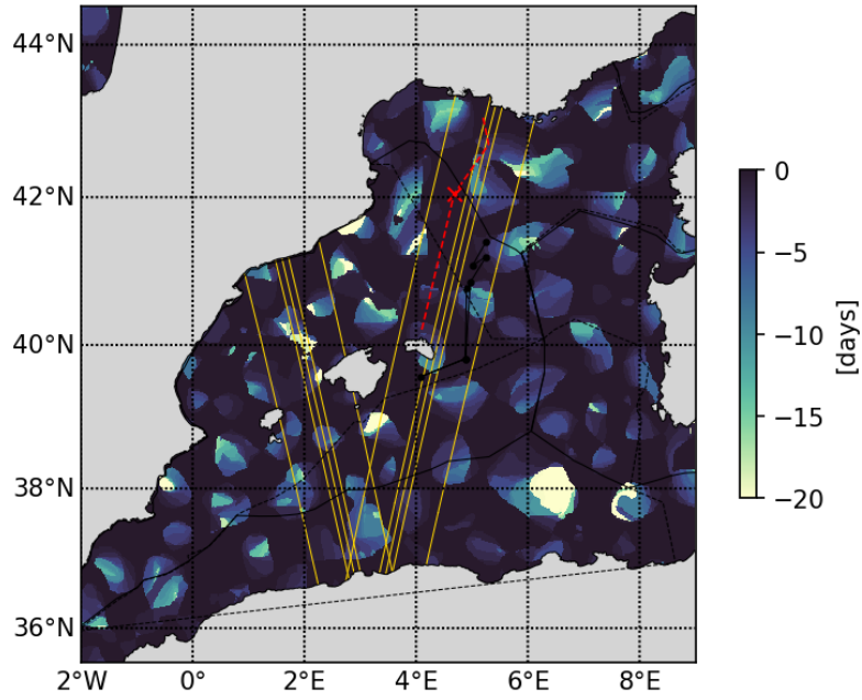
20230507 Retention parameter
