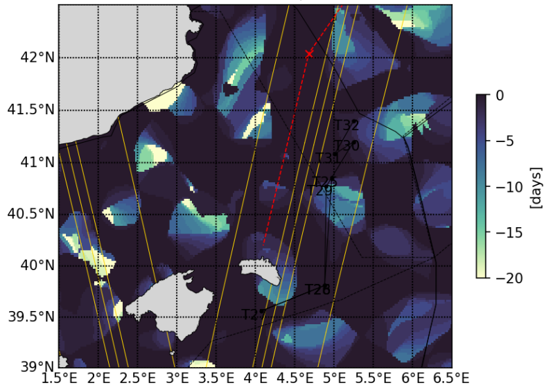
20230507 Retention parameter
