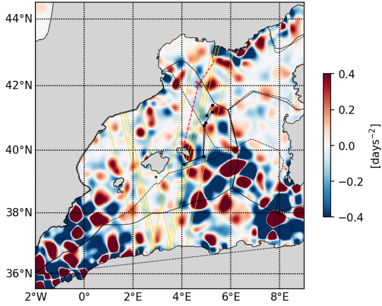
20230507 Okubo-Weiss parameter
