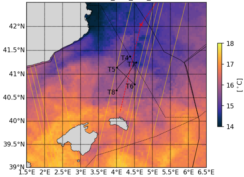
20230424_CLS_SST_7d
