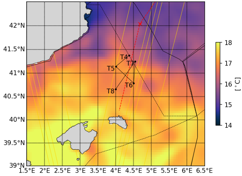
20230425_Copernicus_SST_L4
