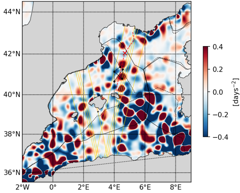
20230426 Okubo-Weiss parameter
