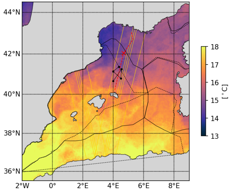
20230424_CLS_SST_7d
