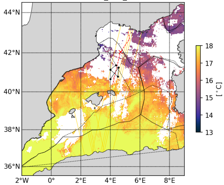
20230425_CLS_SST
