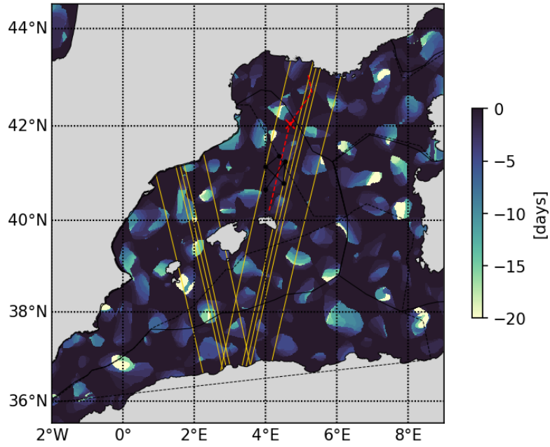
20230426 Retention parameter
