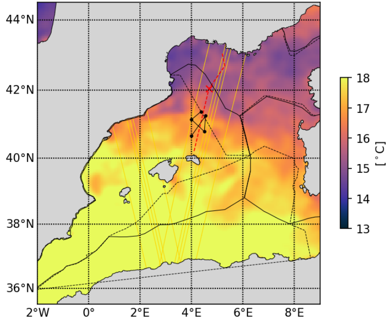
20230425_Copernicus_SST_L4
