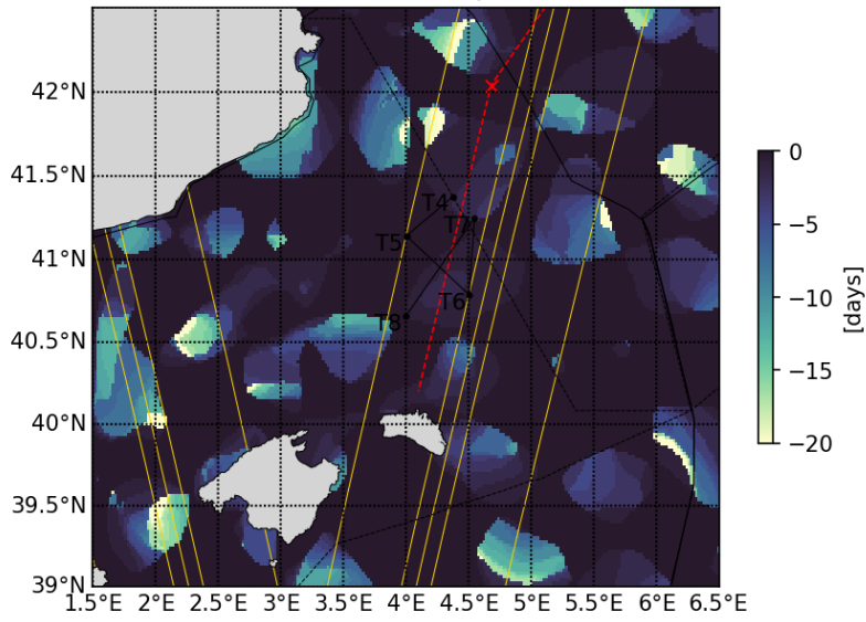
20230426 Retention parameter
