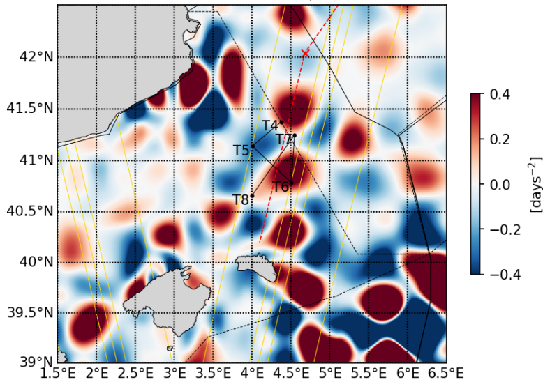
20230426 Okubo-Weiss parameter
