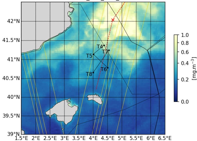
20230425_CLS_CHL_10d
