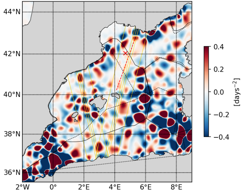
20230417 Okubo-Weiss parameter
