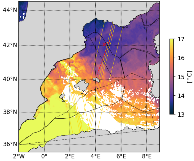
20230416_CLS_SST
