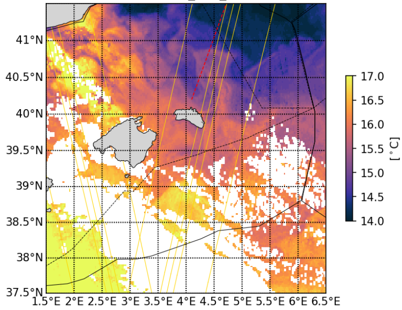
20230416_CLS_SST
