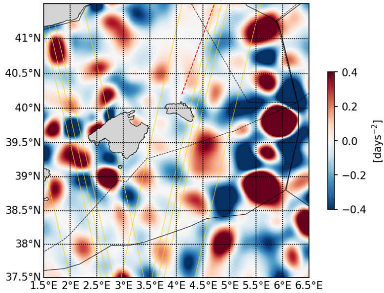
20230417 Okubo-Weiss parameter
