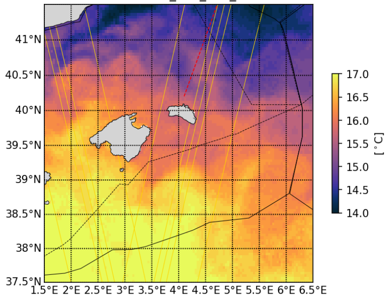
20230415_CLS_SST_7d
