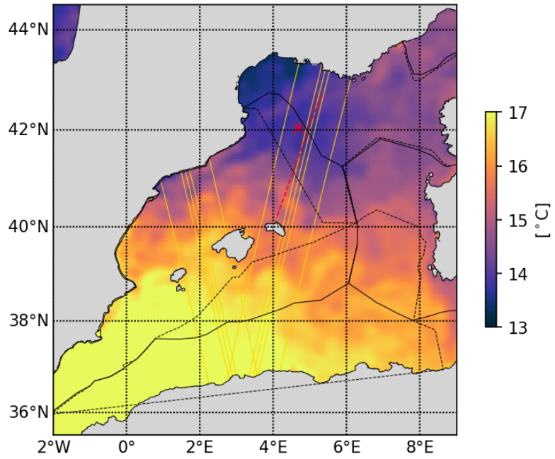
20230416_Copernicus_SST_L4
