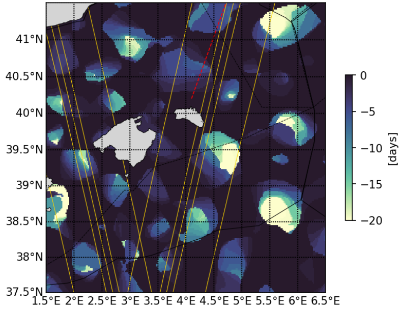
20230417 Retention parameter
