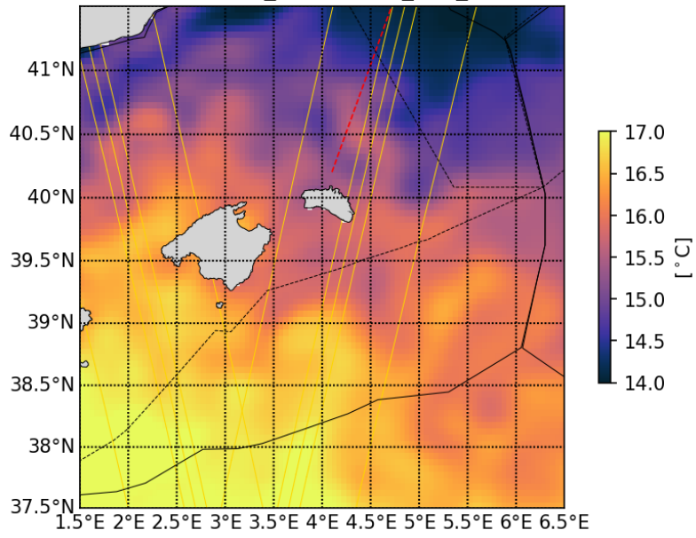
20230416_Copernicus_SST_L4
