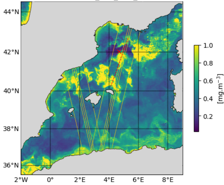
20230309_CLS_CHL_5d
