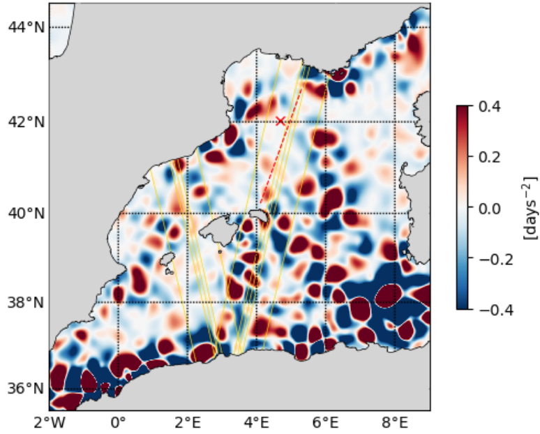
20230312 Okubo-Weiss parameter
