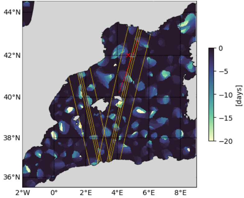
20230312 Retention parameter
