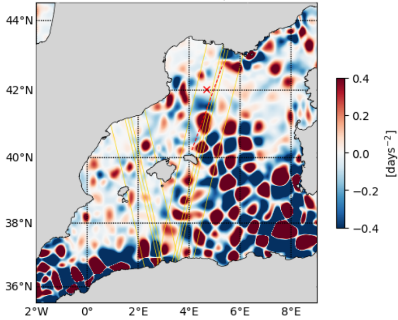
20230302 Okubo-Weiss parameter
